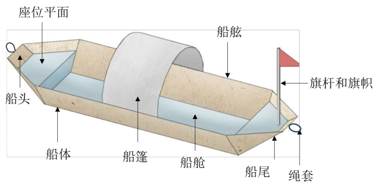
图 3 乌篷船模型示意图
